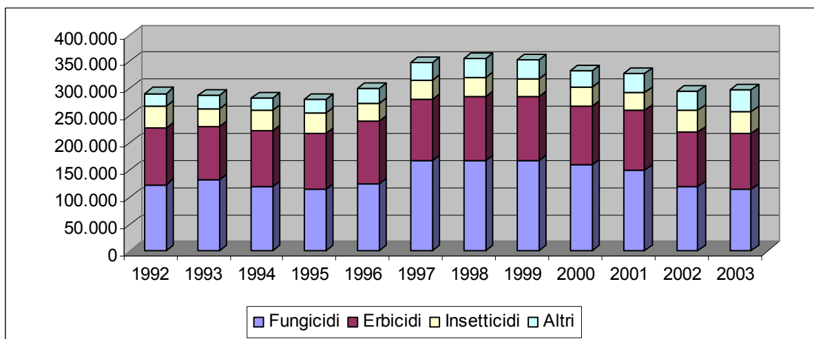
Figura 1: Vendita di sostanze attive dei prodotti fitosanitari (in tonnellate) nell'UE-15
